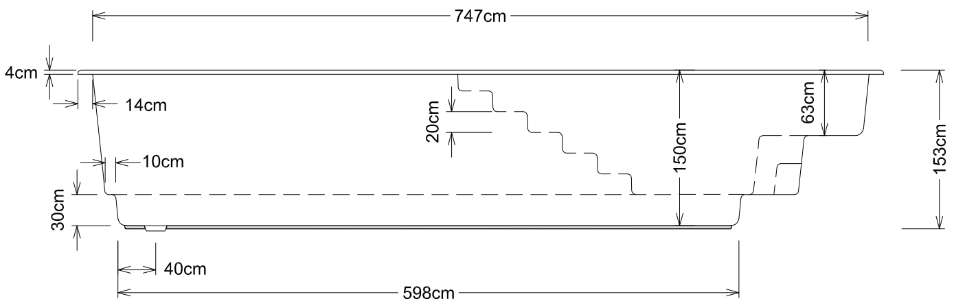
Schnitt - Sezione
