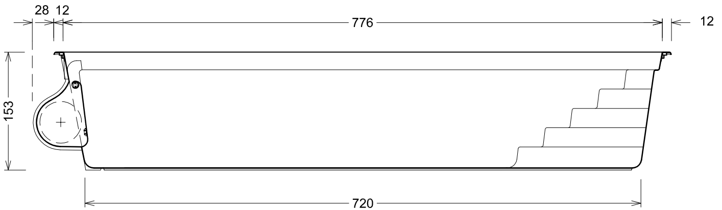
Längsschnitt - longitudinal section
