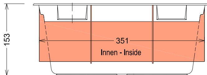
Ansicht Skimmerseite - View skimmer side
