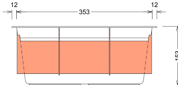
Ansicht Skimmerseite - View skimmer side
