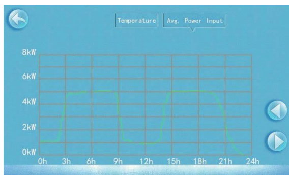
Anzeige durchschnittlicher Stromaufnahme
