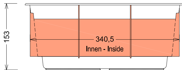
Ansicht Skimmerseite - View skimmer side
