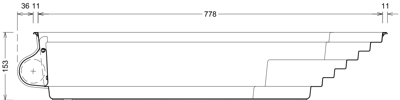
Längsschnitt - longitudinal section
