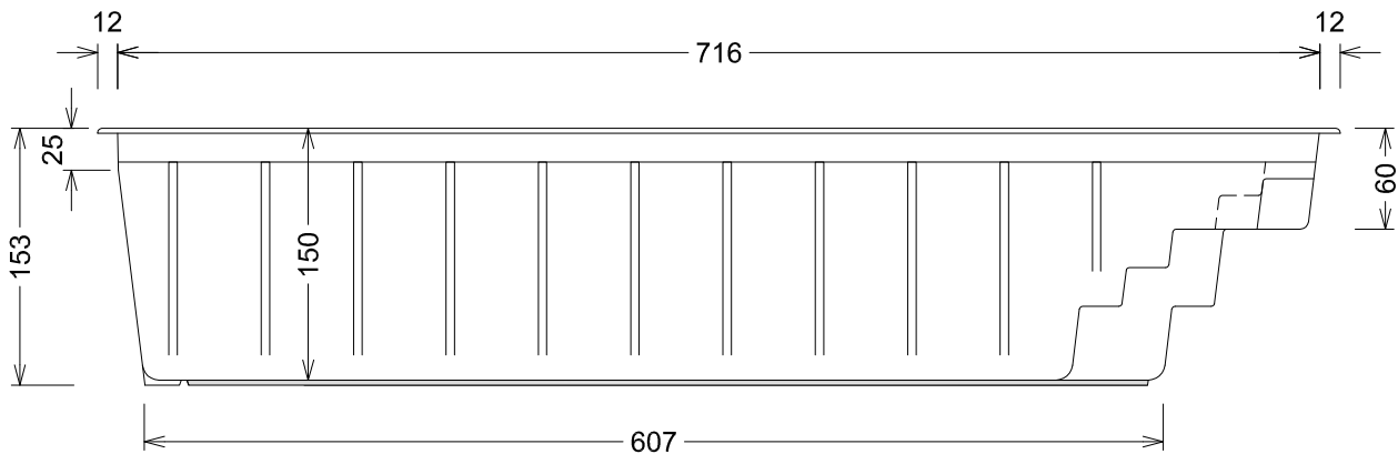
Seitenansicht - Side view
