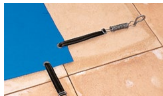
STAR: Gurt + Dynamometerfedern & Kunststoffösen
